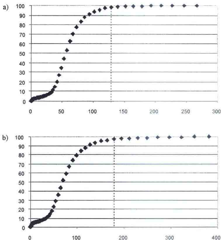
Rys. 4. Dystrybuanty empiryczne rozkładu wielkości ziarn uzyskane laserowym miernikiem wielkości cząstek (IPS): a) dla diabazu (klasa 0,04\pm 0,063 mm); b) dla magnezytu (klasa 0,063\pm 0,071 mm)
