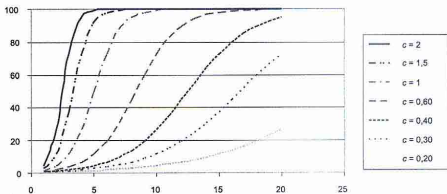
Rys. 3. Kształty dystrybuant rozkładu logistycznego przy różnych wartościach parametru c
