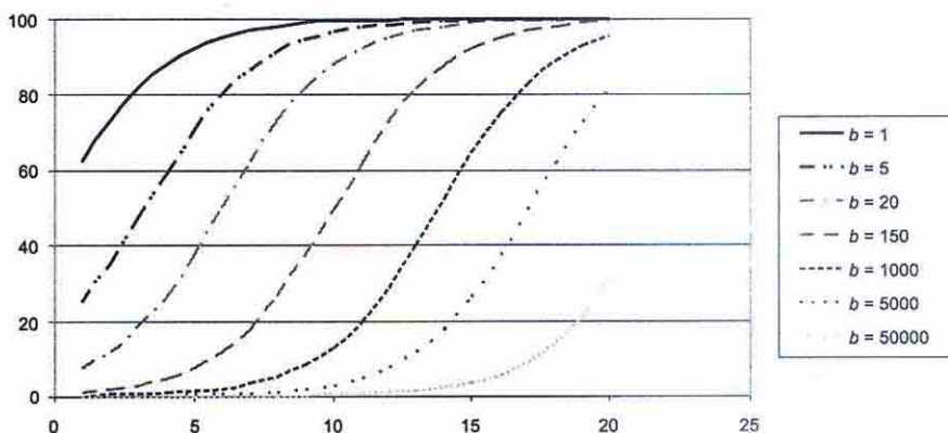
Rys. 2. Kształty dystrybuant rozkładu logistycznego przy różnych wartościach parametru b
